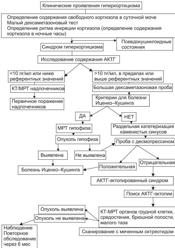
Рис. 14-2. Диагностический алгоритм.
